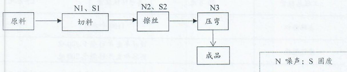
图 2-1 工艺流程及排污节点图
